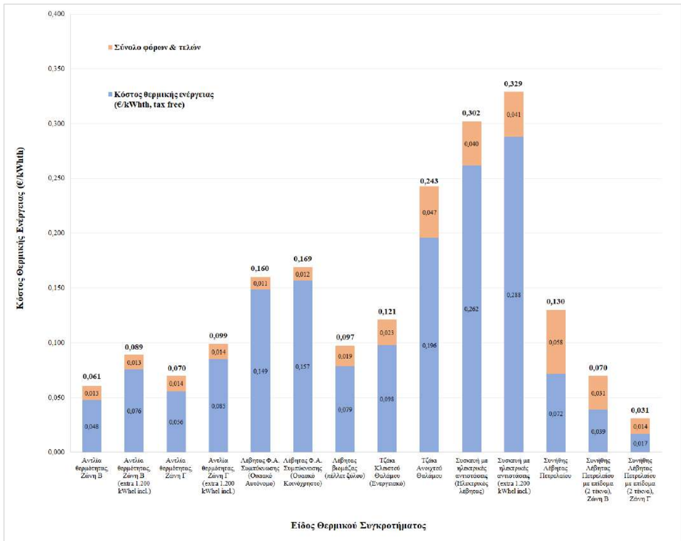
Διάγραμμα 1: Κόστος ωφέλιμης θερμικής ενέργειας ανά είδος θερμικού συγκροτήματος (μέσο νοικοκυριό με θερμικές ανάγκες περί τις 3.000 kWh th /4μνη ή ισοδύναμα 4.500 kWh th /σεζόν).
