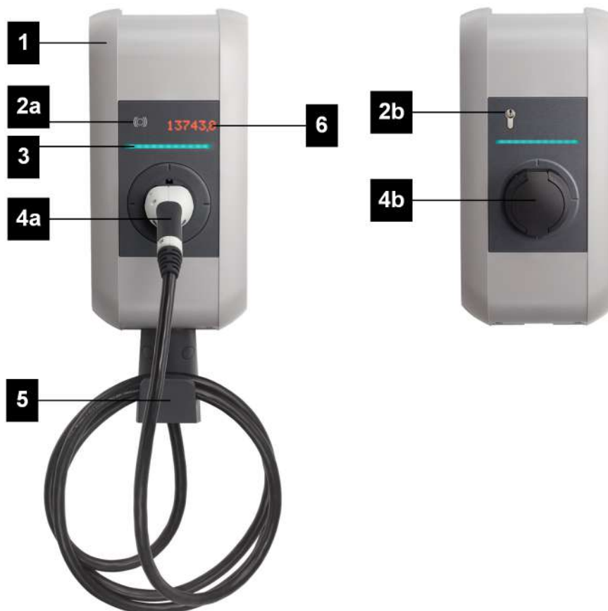
Εικ. 3-1: Επισκόπηση σταθμού φόρτισης
